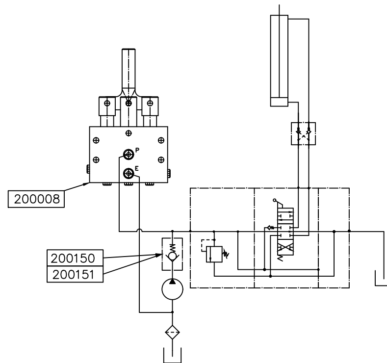
Circuito Hidráulico
