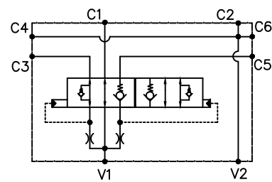
Esquema Hidráulico
