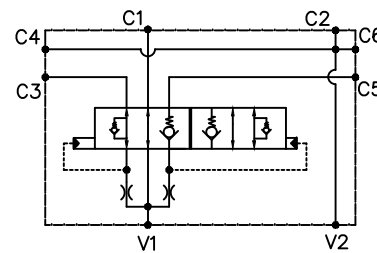
Esquema Hidráulico
